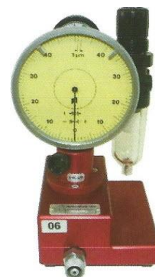
PFL – pneumatisch analog Konverter
